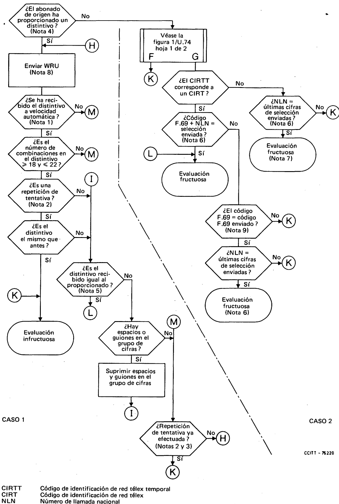
FIGURA 1/U.75 Evaluación del distintivo télex llamado
