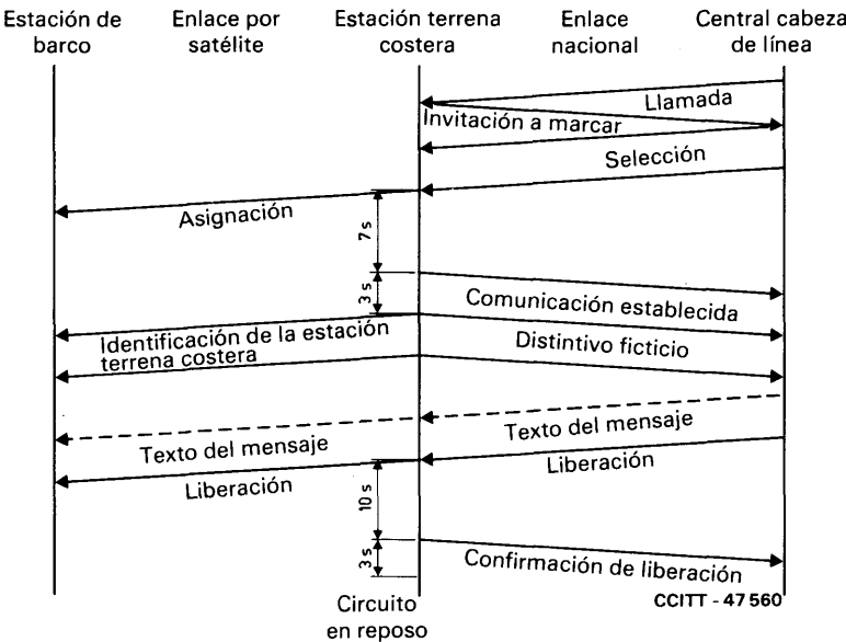
FIGURA 6 Llamada en difusión
