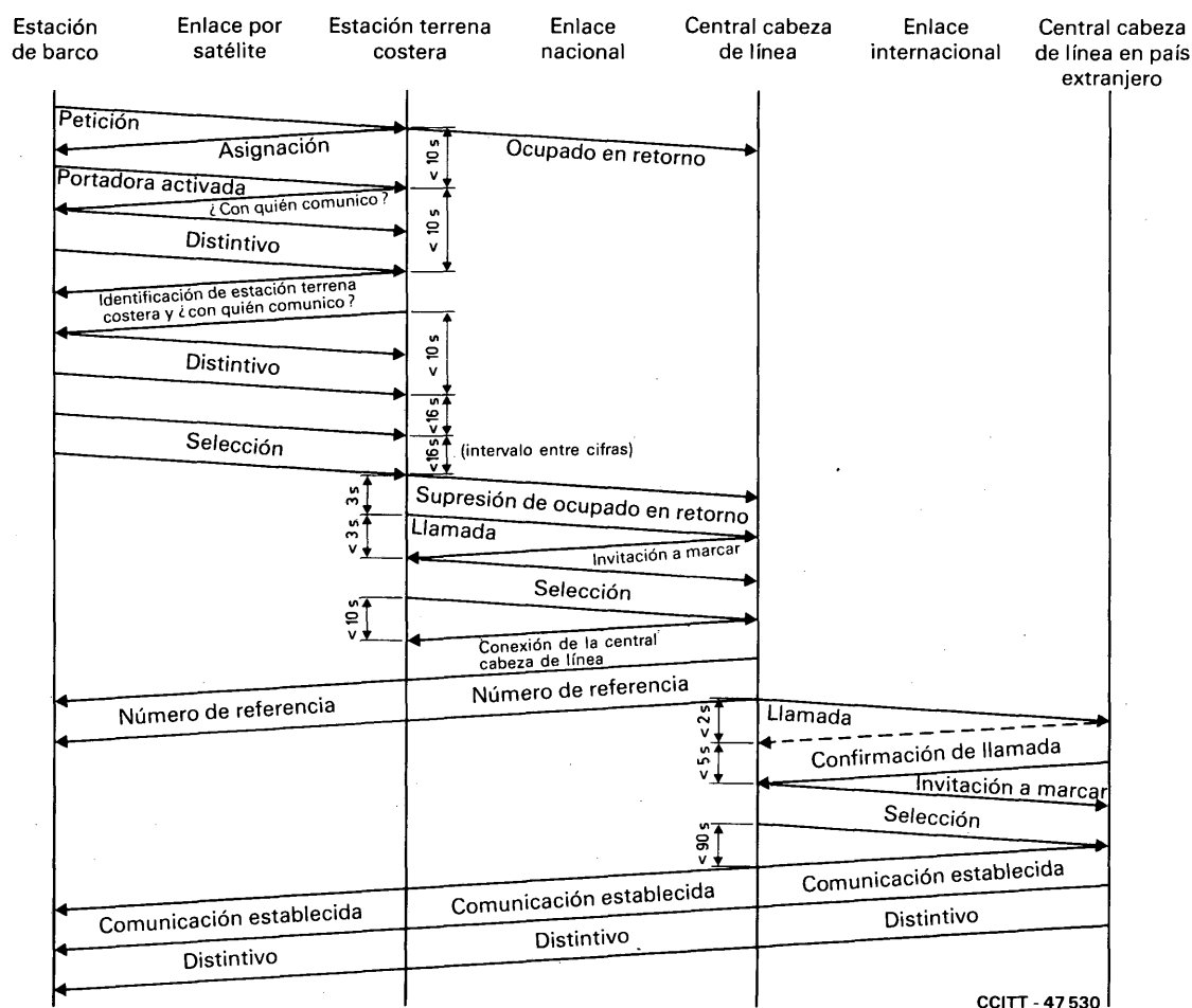
FIGURA 3 Llamada originada en el barco
