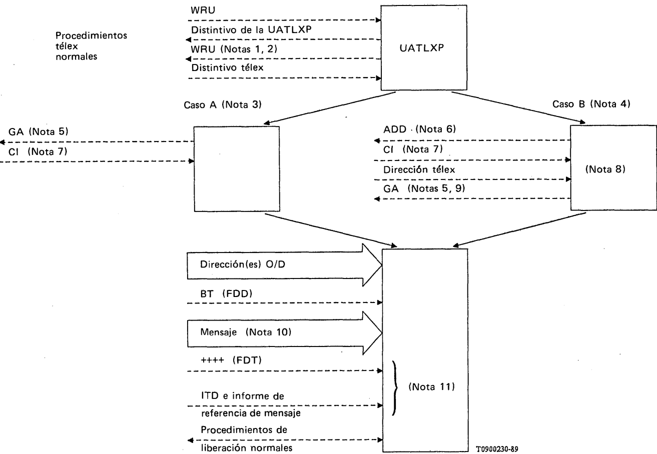
FIGURA 4/U.204 Procedimientos de acceso télex a la UATLXP utilizando la selección en dos etapas (aplicable a un terminal manual o a un DEAT)
