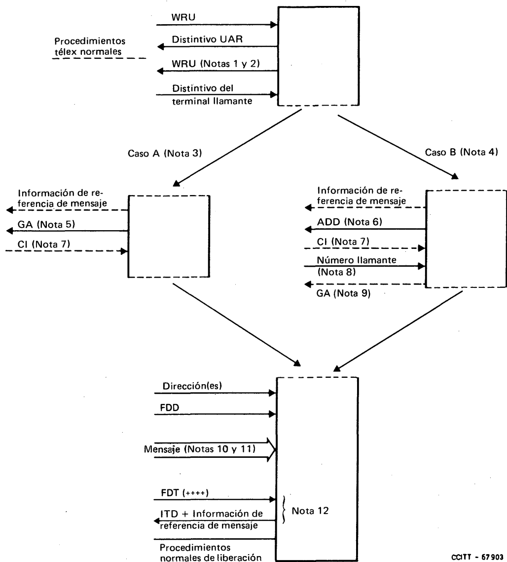
FIGURA 1/U.80 Protocolo de acceso a la unidad de almacenamiento y retransmisión (UAR)
