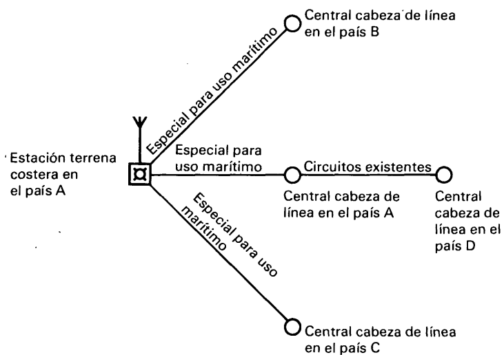
a) Estación terrena costera con funciones de encaminamiento y tarificación
