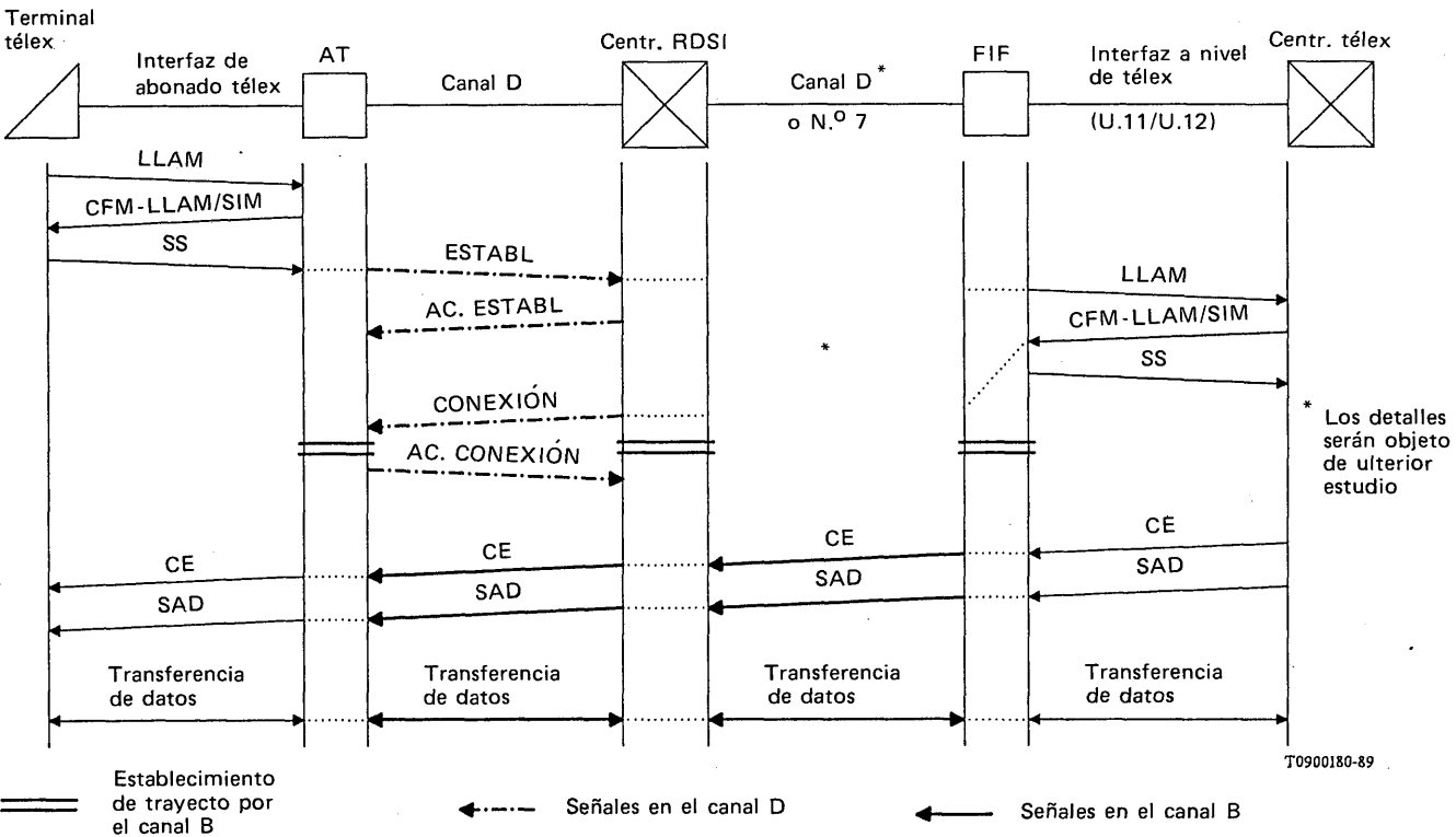
FIGURA 7/U.202 Secuencia de establecimiento de la comunicación en el sentido de la RDSI a la red télex (modelo de integración máxima)
