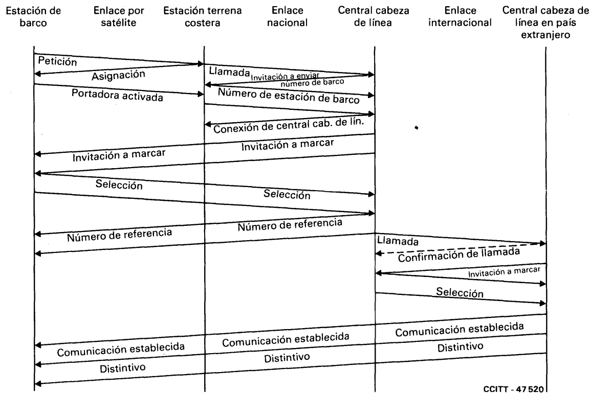
FIGURA 2 Ejemplo de un procedimiento para el establecimiento de la comunicación
