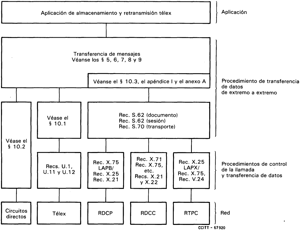
FIGURA 1/U.82 Estructura general de una transferencia de mensajes entre UAR télex
