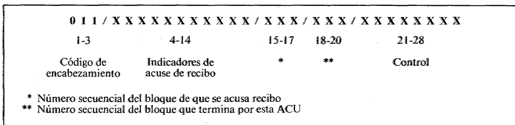
FIGURA 8/Q.259 Formato de la unidad de señalización de acuse de recibo
