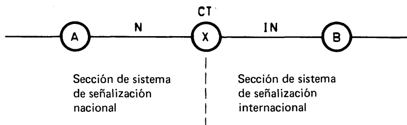
FIGURA 1/Q.300 Punto de interfuncionamiento, ejemplo 1
