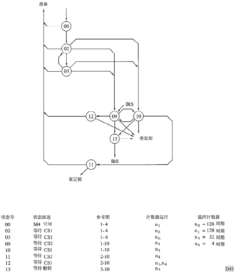
图3/8 在4位信号呼叫标识情况下的无自动识别定相程序（呼叫台） 和电台处于ISS位置的通信流程（状态概图）
