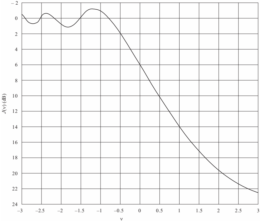
刀刃形障碍物绕射损耗
