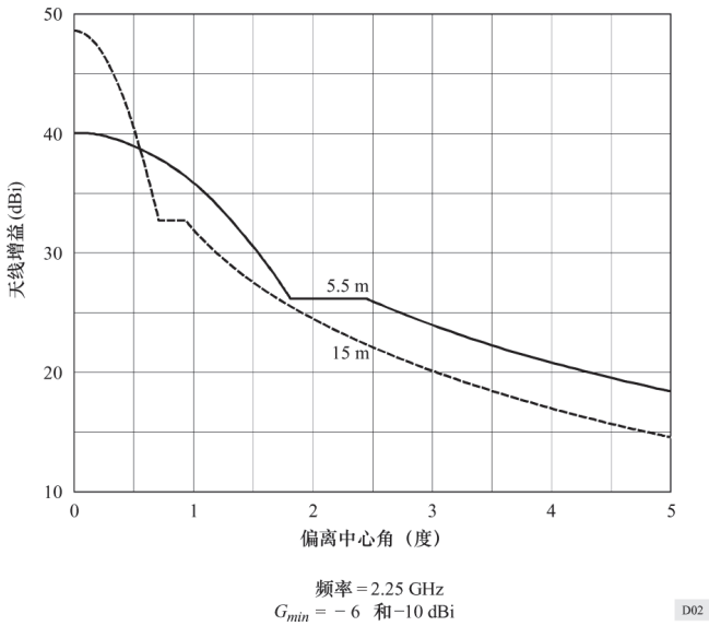
卫星地球站的典型天线特性
