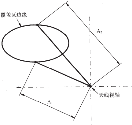
a) 覆盖区外的视轴
