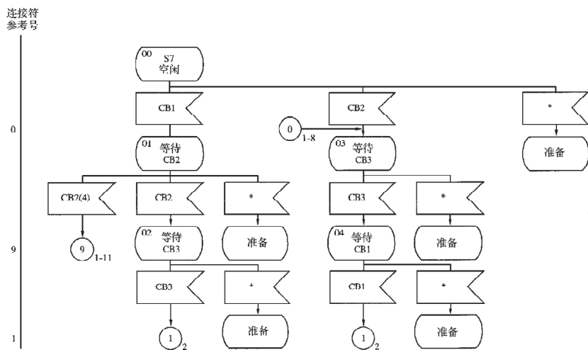
图1/3 在7位信号呼叫标识情况下的自动识别定相程序（被呼叫台）
