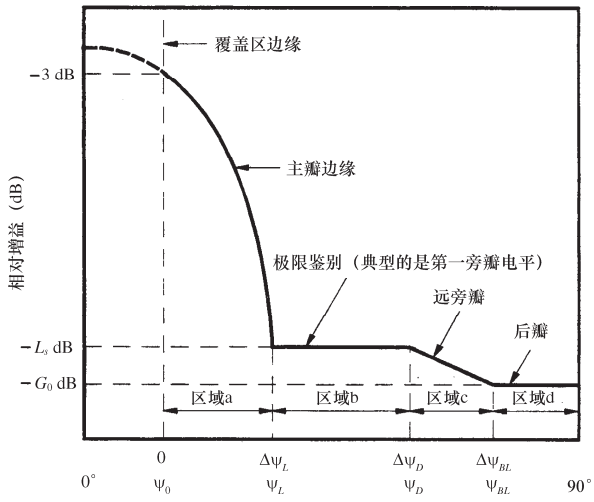
图 2 基准辐射方向图的可能形状
