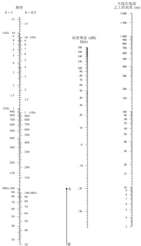
图6 圆形地球上的绕射 - 天线高度增益
