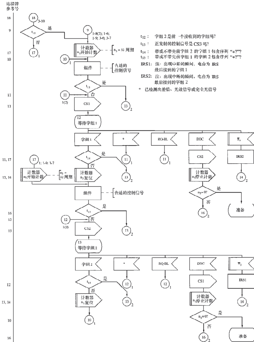
图1/2 在4位信号呼叫标识和7位信号呼叫标识情况下的通信流程（电台处于IRS位置）
