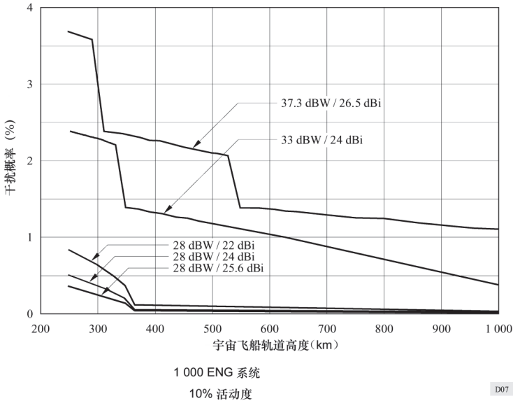
图 7 各种 ENG 系统特性的干扰概率
