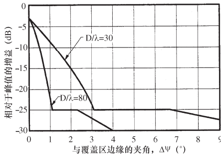
图 6 建议的中等扫描比( 3.5 < \delta < 5.0 )的基准方向图
