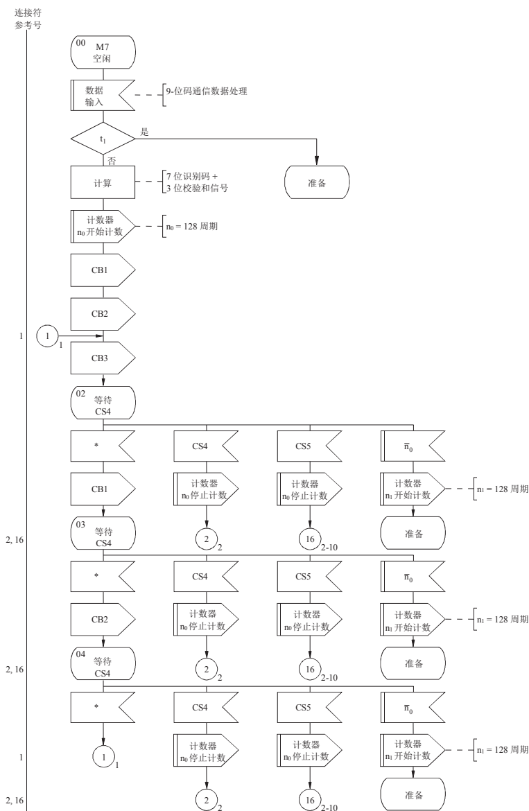
图1/3 在7位信号呼叫标识情况下的自动识别定相程序（呼叫台）
