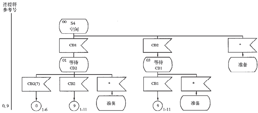
图1/1 在4位信号呼叫标识情况下的无自动识别定相程序（被呼叫台）
