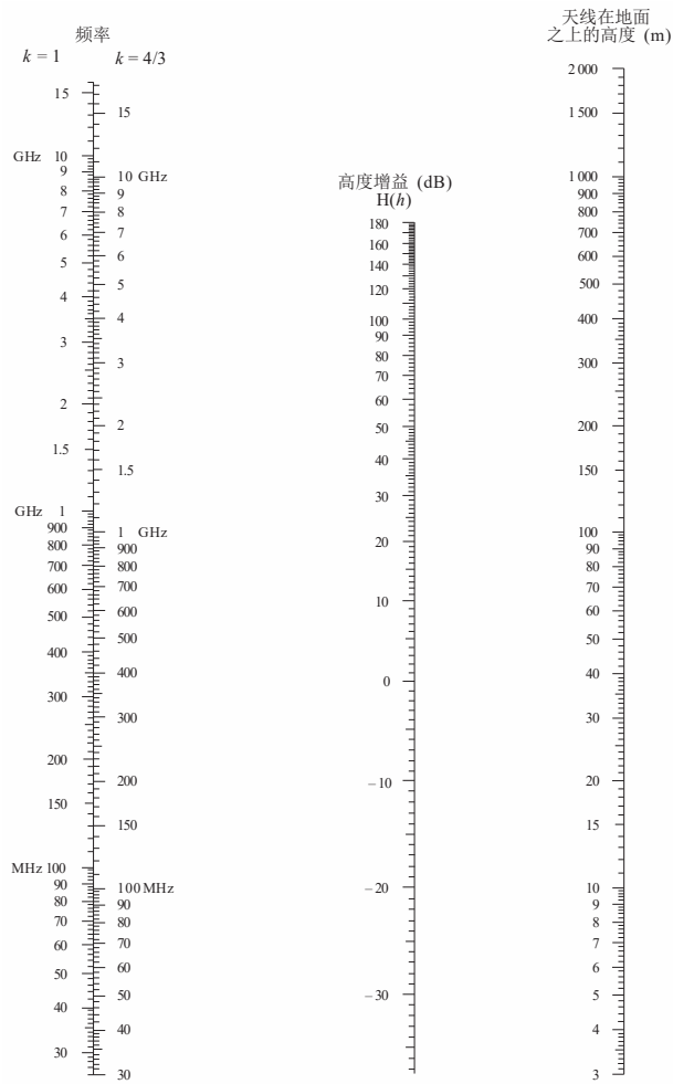
圆形地球上的绕线 - 天线高度增益
