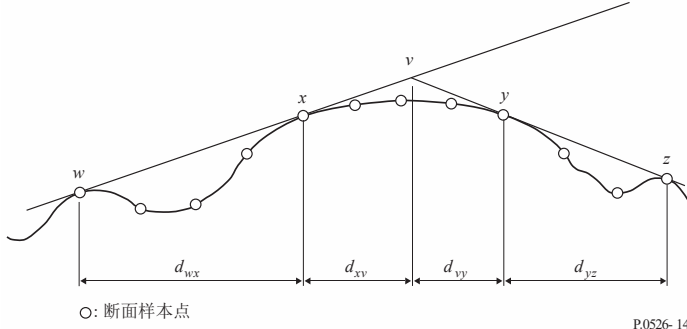
图14 多点障碍物的几何图
