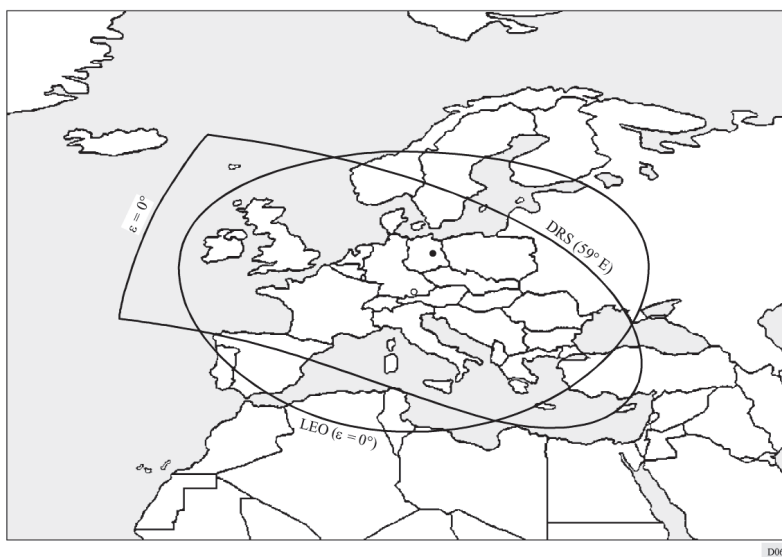
图 6 数据中继卫星天线和 250 km LEO 的覆盖范围
