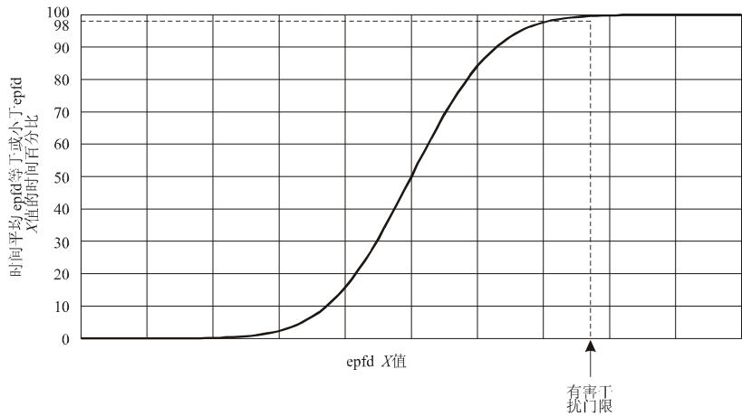
图 2 一个单元的累计等效功率通量密度分布的举例
