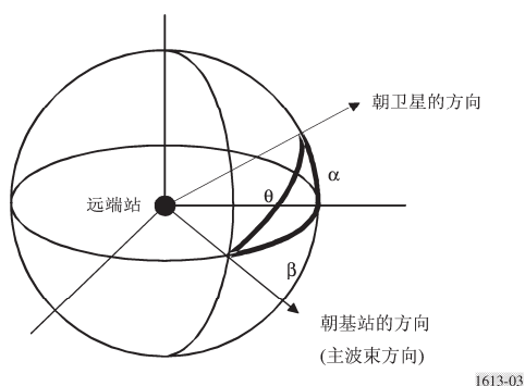
远端站朝向 EESS/SRS 卫星的偏轴角 \theta
