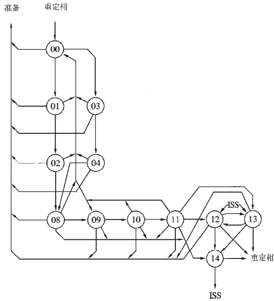
图6/8 在7位信号呼叫标识情况下的自动识别重定相程序（被呼叫台） 和电台处于IRS位置的通信流程（状态概图）
