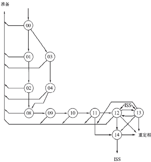
图5/8 在7位信号呼叫标识情况下的自动识别定相程序（被呼叫台） 和电台处于IRS位置的通信流程（状态概图）
