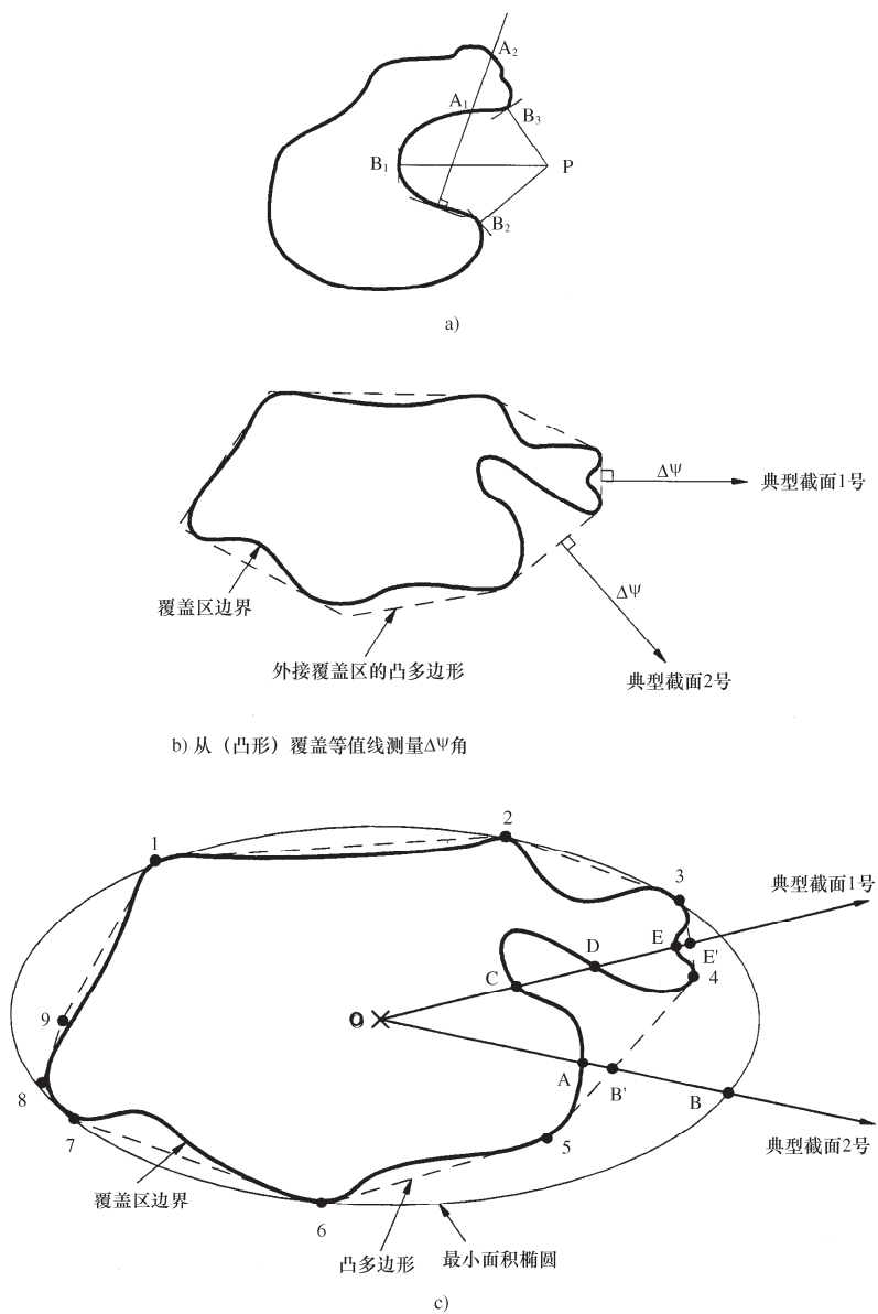
图 3 覆盖区的各种表示法
