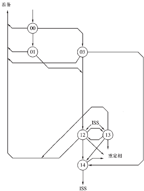
图7/8 在4位信号呼叫标识情况下的无自动识别定相程序（被呼叫台） 和电台处于IRS位置的通信流程（状态概图）
