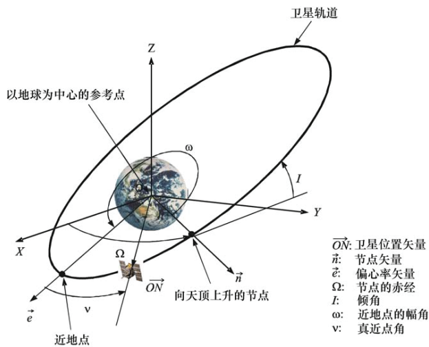
图 3 坐标中的椭圆轨道几何图
