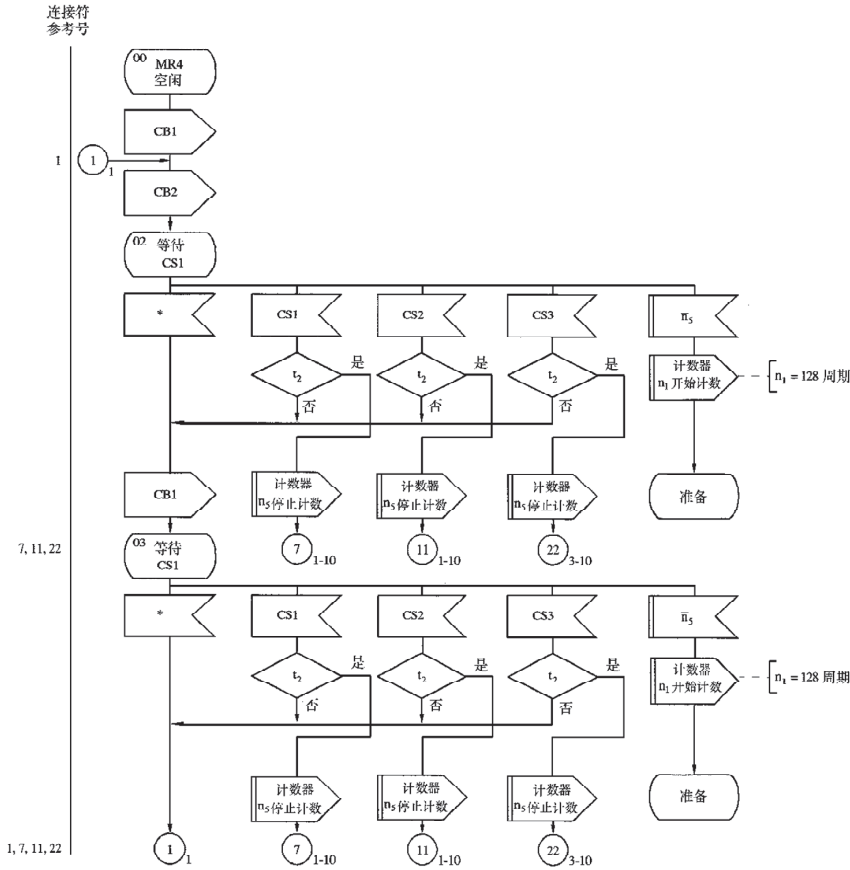
图1/1 在4位信号呼叫标识情况下的无自动识别重定相程序（呼叫台）
