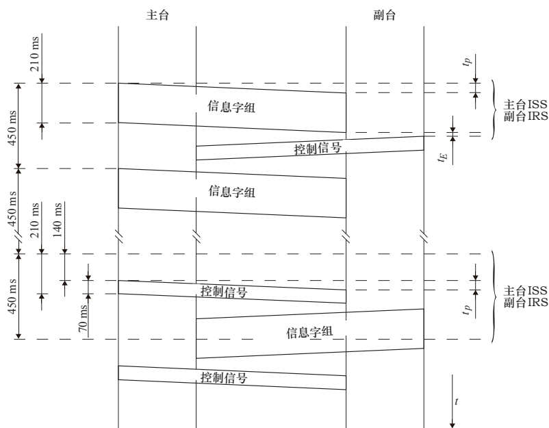
图 1 基本时序图
