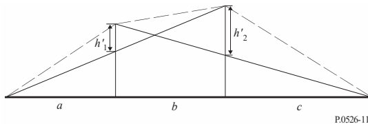
图形11 双重孤立的刀刃形障碍
