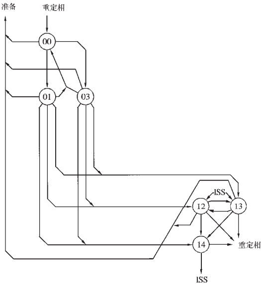
图8/8 在4位信号呼叫标识情况下的无自动识别重定相程序（被呼叫台） 和电台处于IRS位置的通信流程（状态概图）
