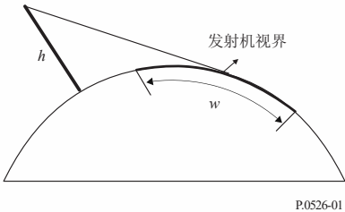
图1 半阴影宽度的确定
