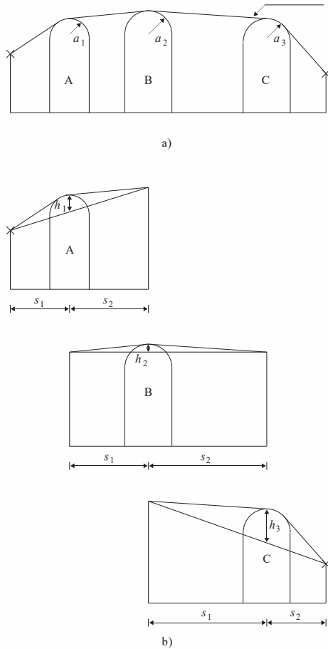
图13 级联圆柱体模型：a) 全部问题；b) 细节
