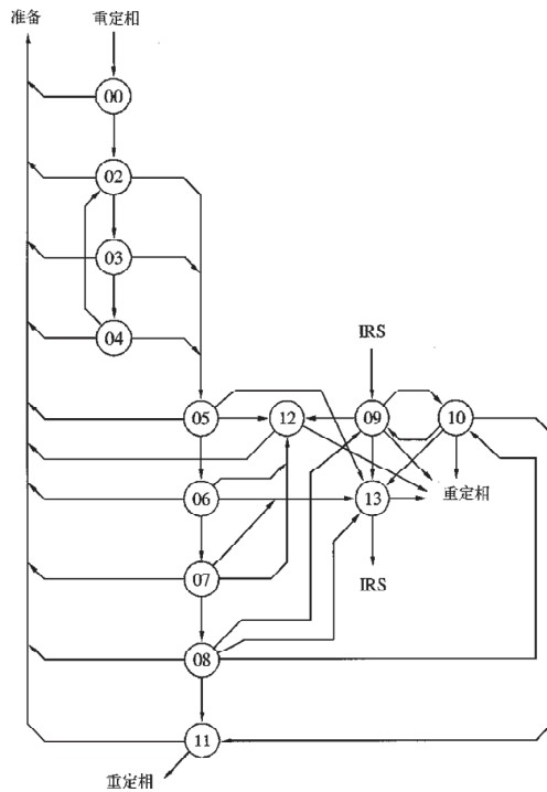
图2/8 在7位信号呼叫标识情况下的自动识别重定相程序（呼叫台） 和电台处于ISS位置的通信流程（状态概图）
