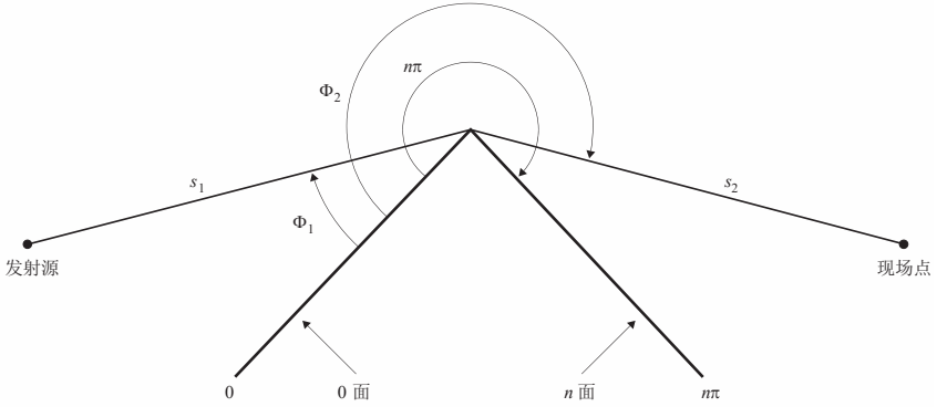
图16 UTD楔绕射场合的集合图
