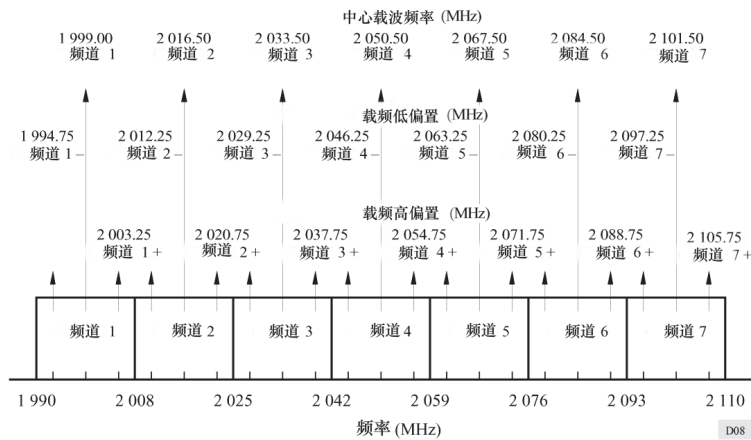
图 8 美国在用的 ENG 频道规划
