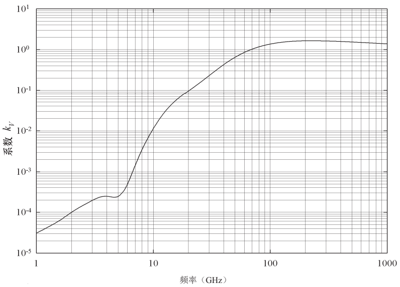
图 3 垂直极化的系数 k_V
