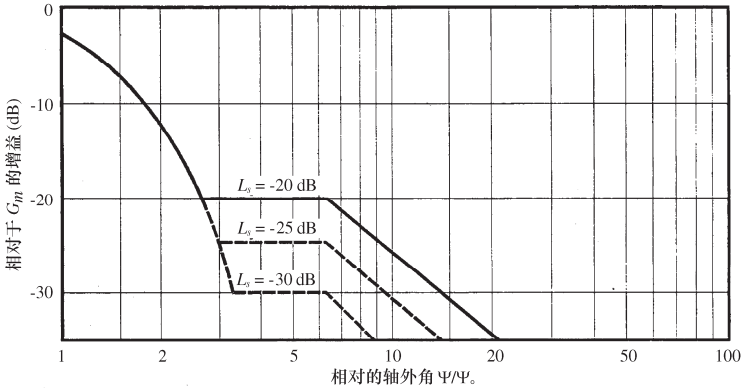
图 1 辐射方向图包络函数
