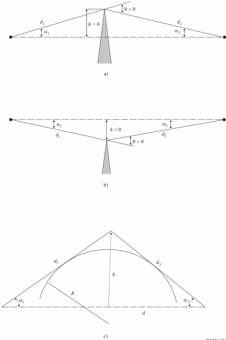
图8 几何参数
