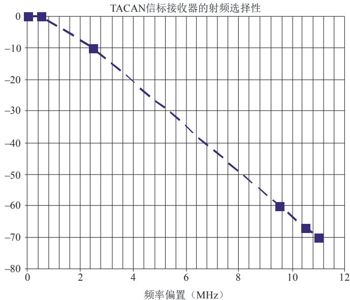
图 2 地面电台（信标）接收器的射频选择性曲线
