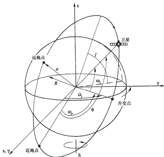
图 4 非 GSO 轨道和参照系
