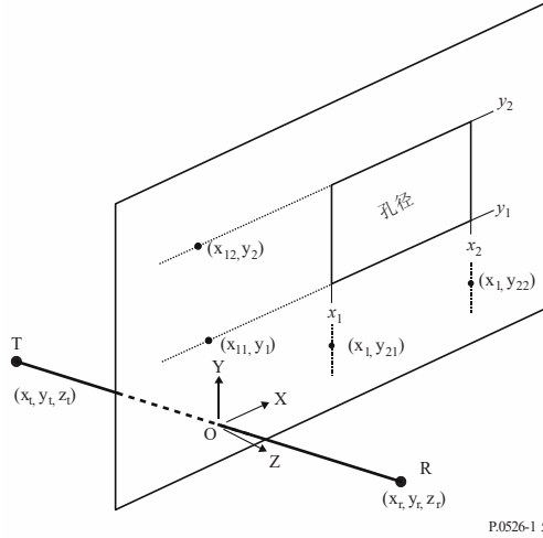
图15 单个矩形孔径的几何图
