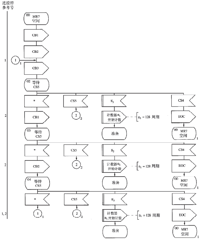
图1/3 在7位信号呼叫标识情况下的自动识别重定相程序（呼叫台）
