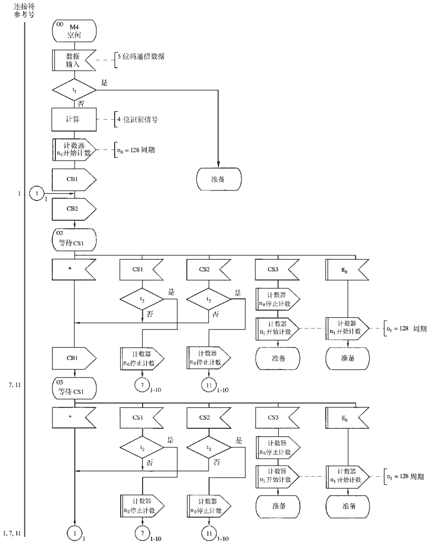
图1/1 在4位信号呼叫标识情况下的无自动识别定相程序（呼叫台）
