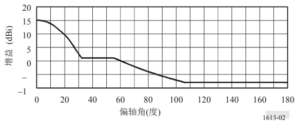
图 2 远端站天线辐射方向性图
