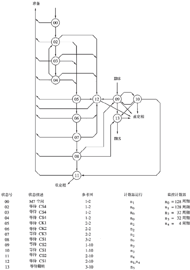
图1/8 在7位信号呼叫标识情况下的自动识别定相程序（呼叫台） 和电台处于ISS位置的通信流程（状态概图）
