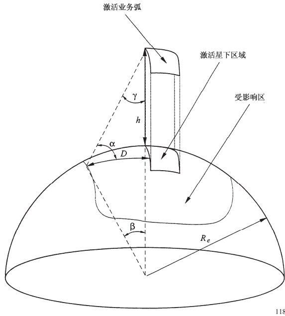
图2 计算星下区域周围包络距离D所需的几何图形
