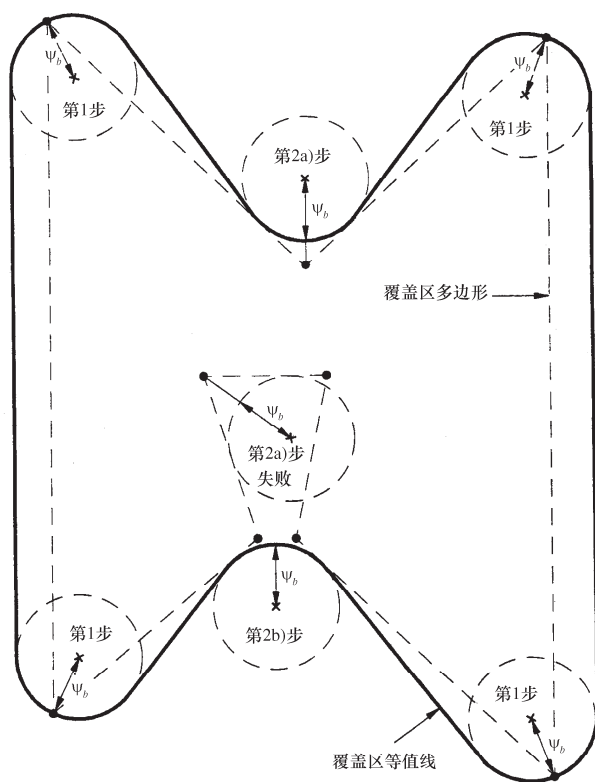
图 7 覆盖区等值线的绘制
