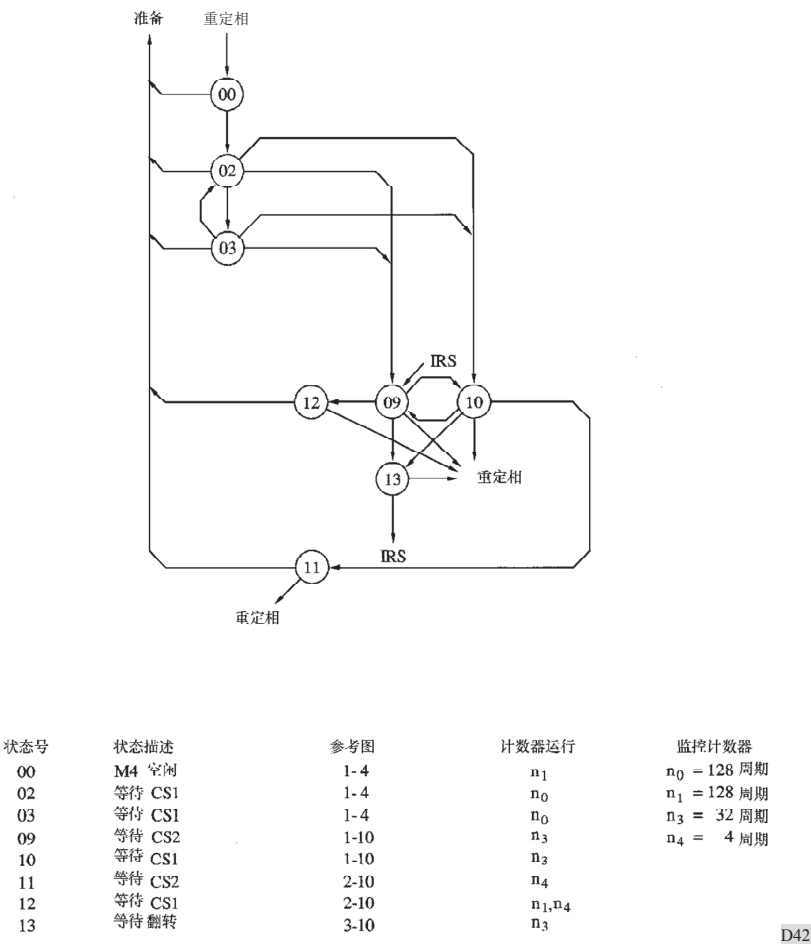
图4/8 在4位信号呼叫标识情况下的无自动识别重定相程序（呼叫台） 和电台处于ISS位置的通信流程（状态概图）
