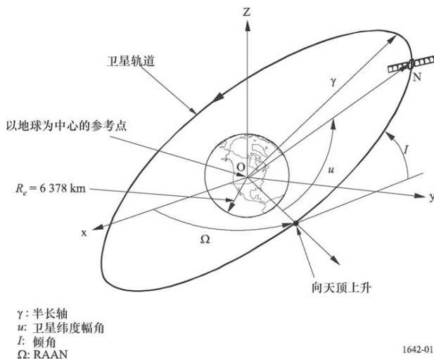
图 1 圆形轨道几何图
