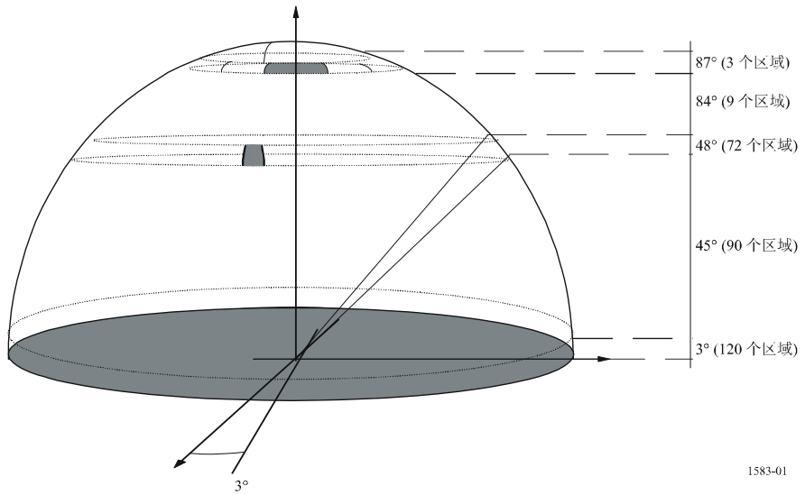
图 1 将天空分为约9平方度的立体角之例
