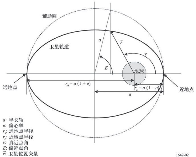
图 2 聚焦平面中椭圆轨道几何图
