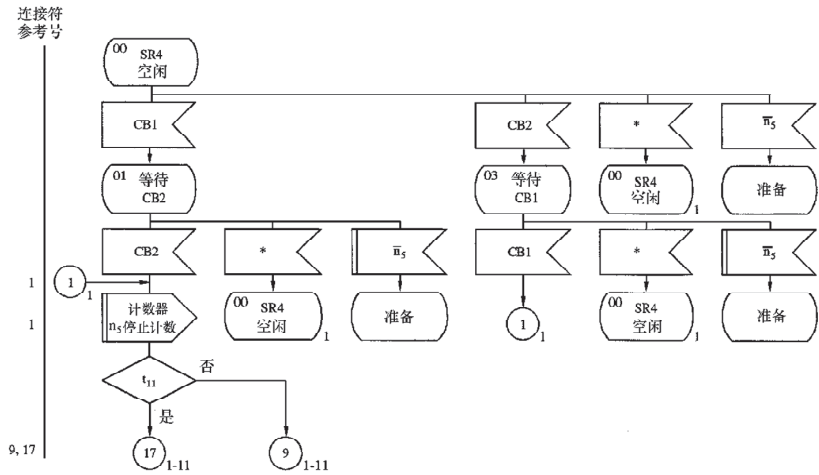
图1/1 在4位信号呼叫标识情况下的无自动识别重定相程序（被呼叫台）
