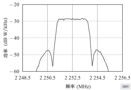
图 9 频谱样例
