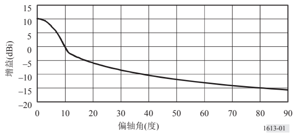
基站天线辐射图
