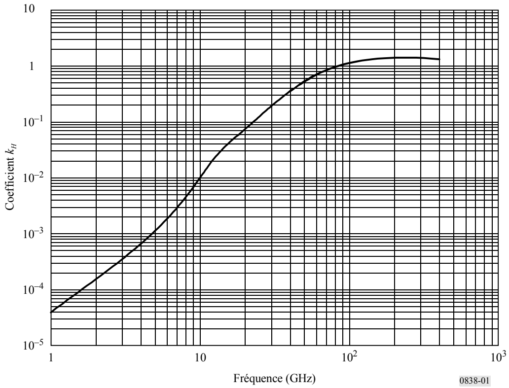
Variation de k en fonction de la fréquence, en polarisation horizontale
