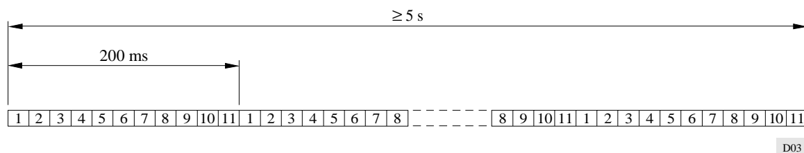
FIGURE 3 Composition du signal d'appel «à tous les navires»
