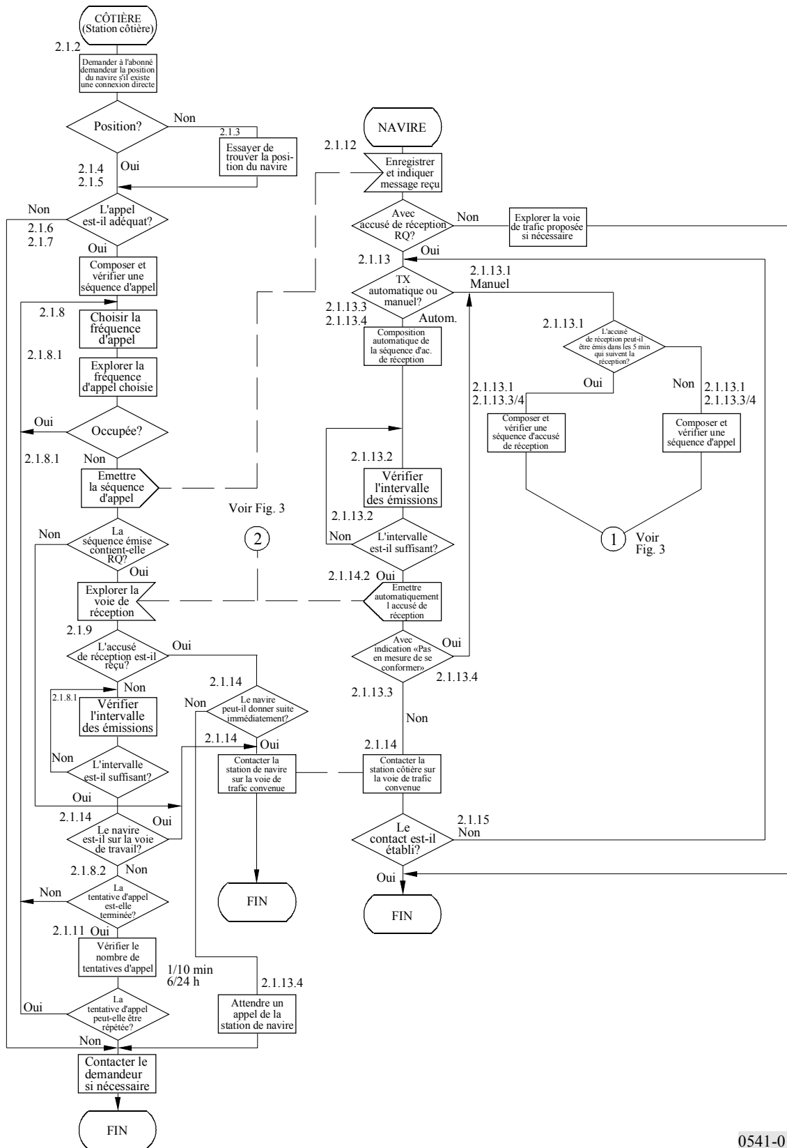
FIGURE 1 Organigramme des procédures d'exploitation pour l'appel dans le sens côtère-navire
