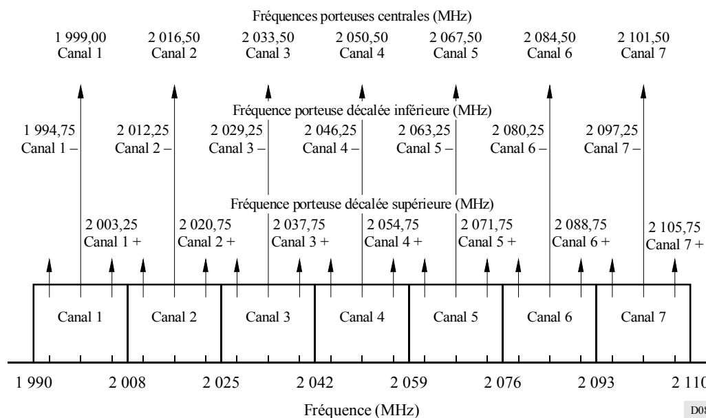
FIGURE 8 Plan des canaux ENG en usage aux Etats-Unis d'Amérique
