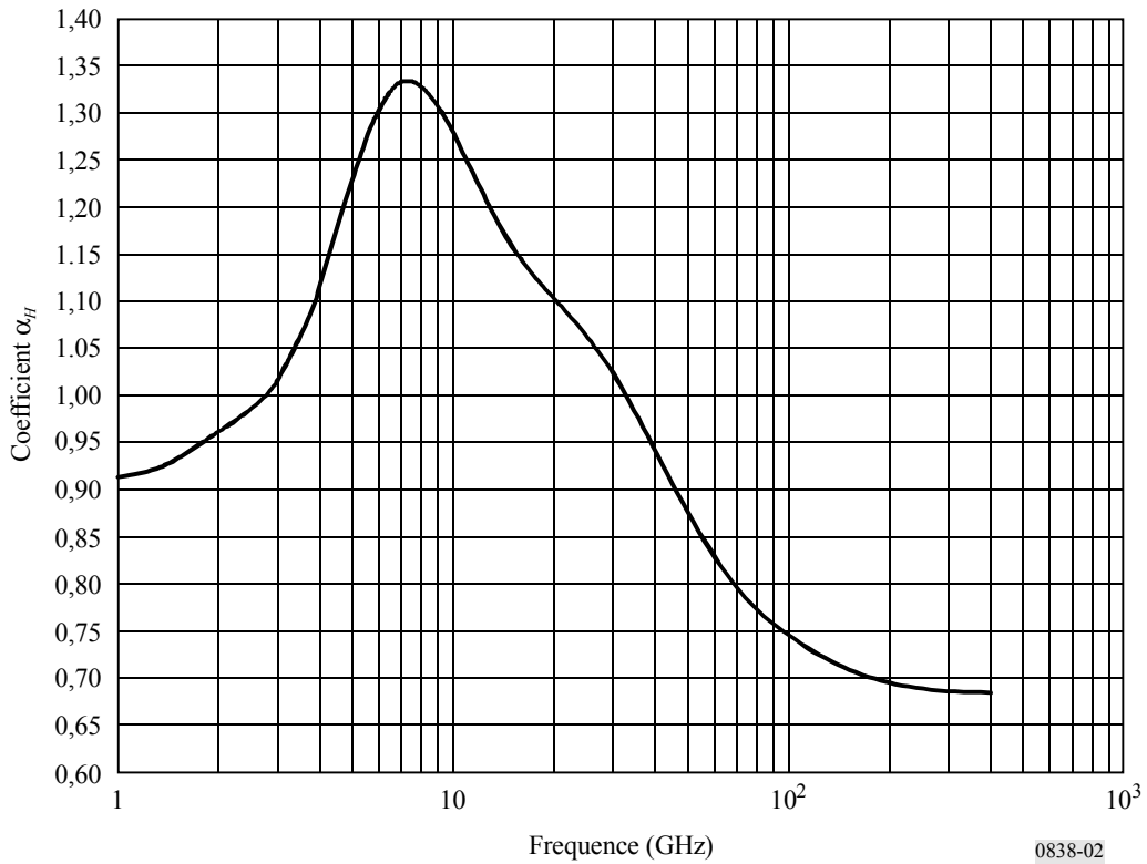
Variation de \alpha en fonction de la fréquence, en polarisation verticale
